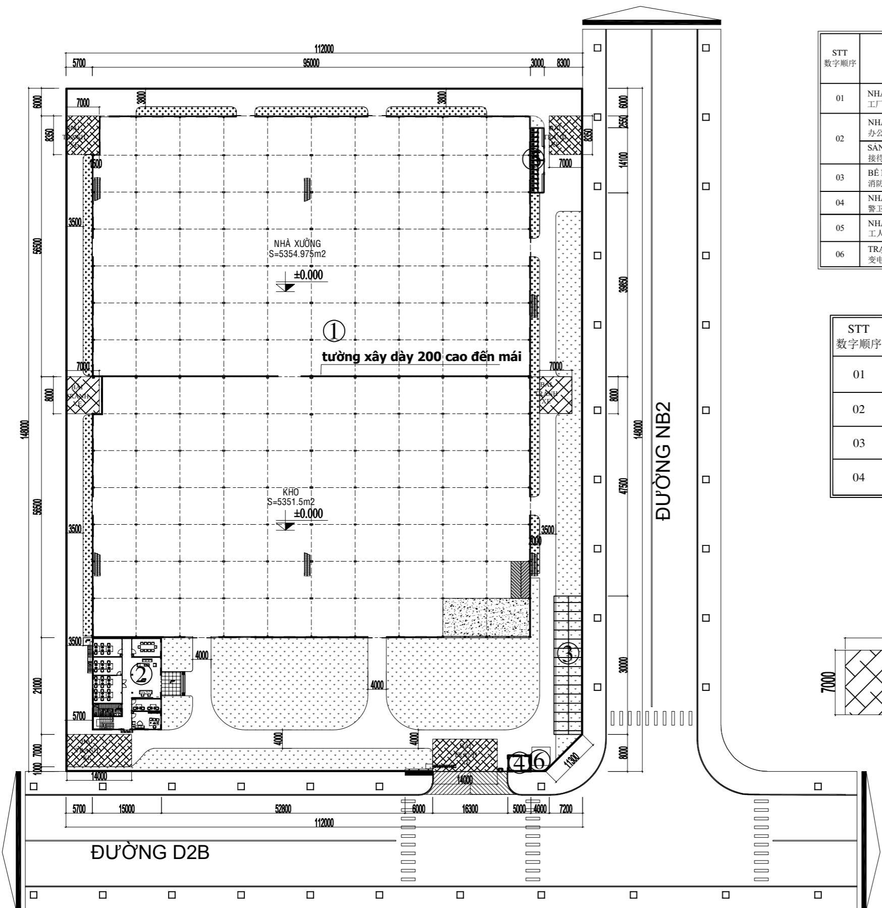
MẶT BẰNG TỔNG THỂ TẦNG 1 TỈ LỆ 1/500
